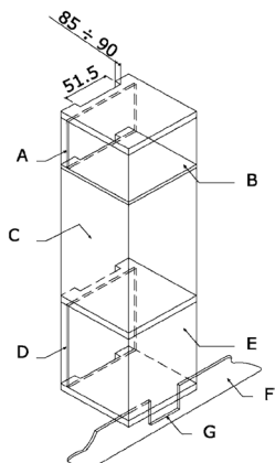
Fig. 8: Conditions requises de ventilation et de découpe pour l'installation d'un four électrique simple dans une armoire haute.
