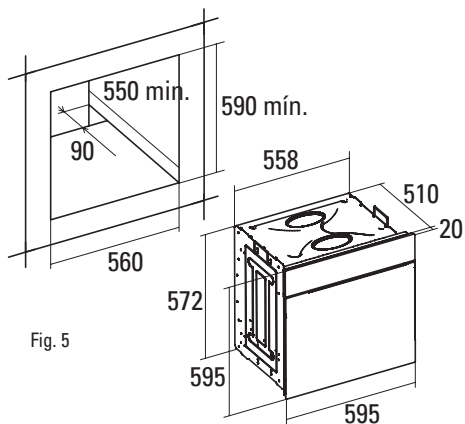
Fig. 5: Distances d'installation pour fours électriques simples de 60 cm de largeur (la forme de la carcasse supérieure peut varier) et de sa fixation dans l'armoire.,
