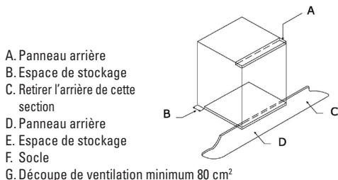
Fig. 8: Conditions requises de ventilation et de découpe pour l'installation d'un four électrique simple dans une armoire haute.
